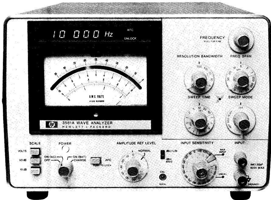
HP 3581A
